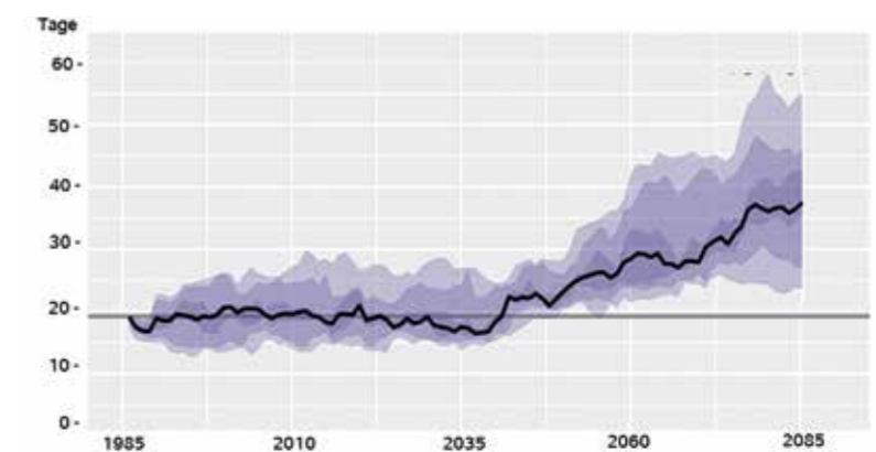
Mittlere Anzahl von Tagen mit Niedrigwasser unter dem Schwellenwert GIQ 1971–2000 für den Pegel Duisburg/Ruhrort (Rhein) im Weiter-wie-bisher-Szenario.
